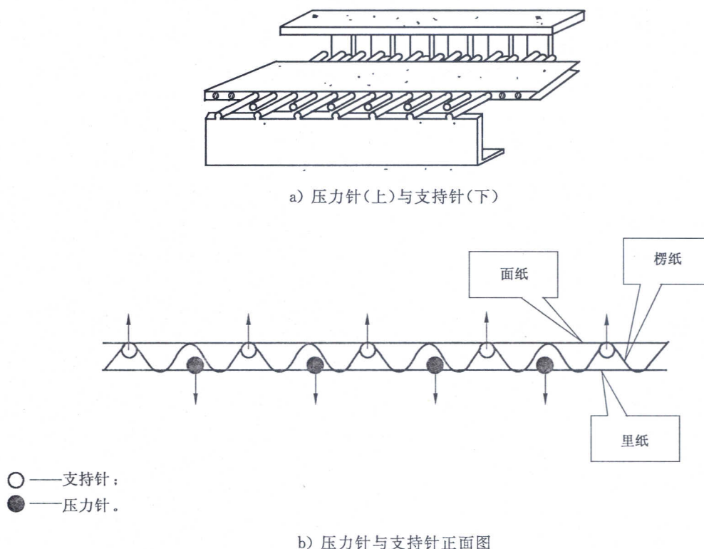
图 2 插针示意图
